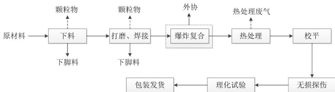
图 2-2 项目工艺流程及产污环节
